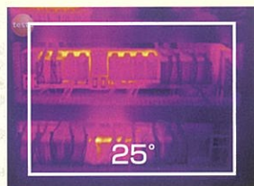
32°(全体)と25°(白枠内)の視野画像の比較
